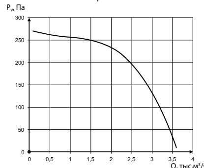
УНИВЕНТ-К1-3,15-4-2
