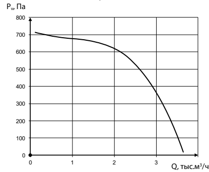
УНИВЕНТ-К1-2,5-2-2
