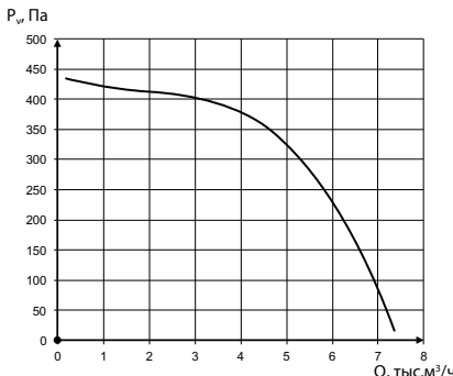
УНИВЕНТ-К1-4-4-2
