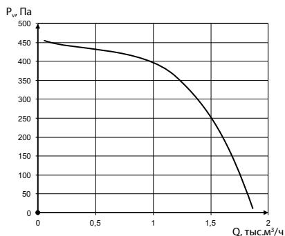
УНИВЕНТ-К1-2-2-2
