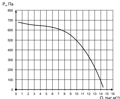
УНИВЕНТ-К1-5-4-2
