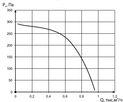
УНИВЕНТ-К1-1,6-2-2
