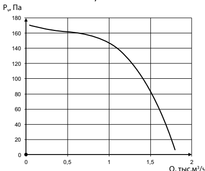
УНИВЕНТ-К1-2,5-4-2
