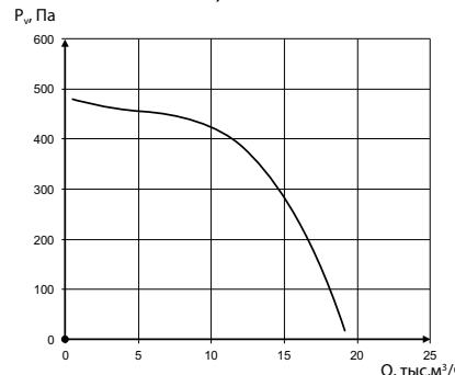
УНИВЕНТ-К1-6,3-6-2
