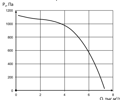
УНИВЕНТ-К1-3,15-2-2
